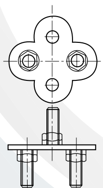
90° Verbindungselement * 1 90° Fastening device Art.Nr.: 220000005
