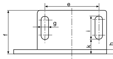
Draufsicht topview
