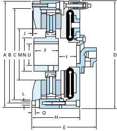
LIM 106 Clutch/Kupplung
