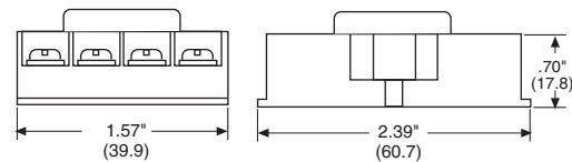
OCTAL SOCKET P/N: 6001-101-001
